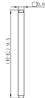
(铜针例图)
