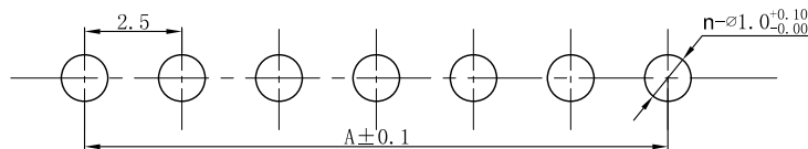
线路板安装尺寸
